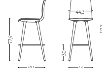
4 wood legs stool without arms Taburete 4 Patas madera sin brazos
