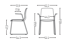
Cantilever with simple arm Patín metálico con brazo simple
